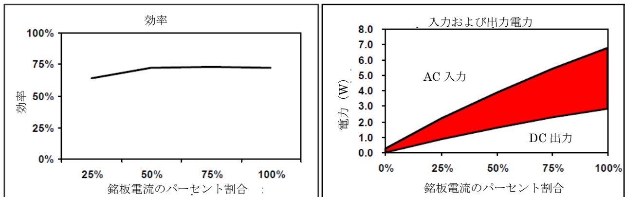
230V50Hz における測定および算出されたデータ
