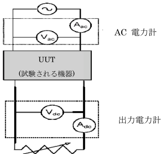
図 2—可変抵抗負荷を使用する一般的試験設定
